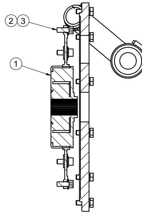
CORTE A-A
